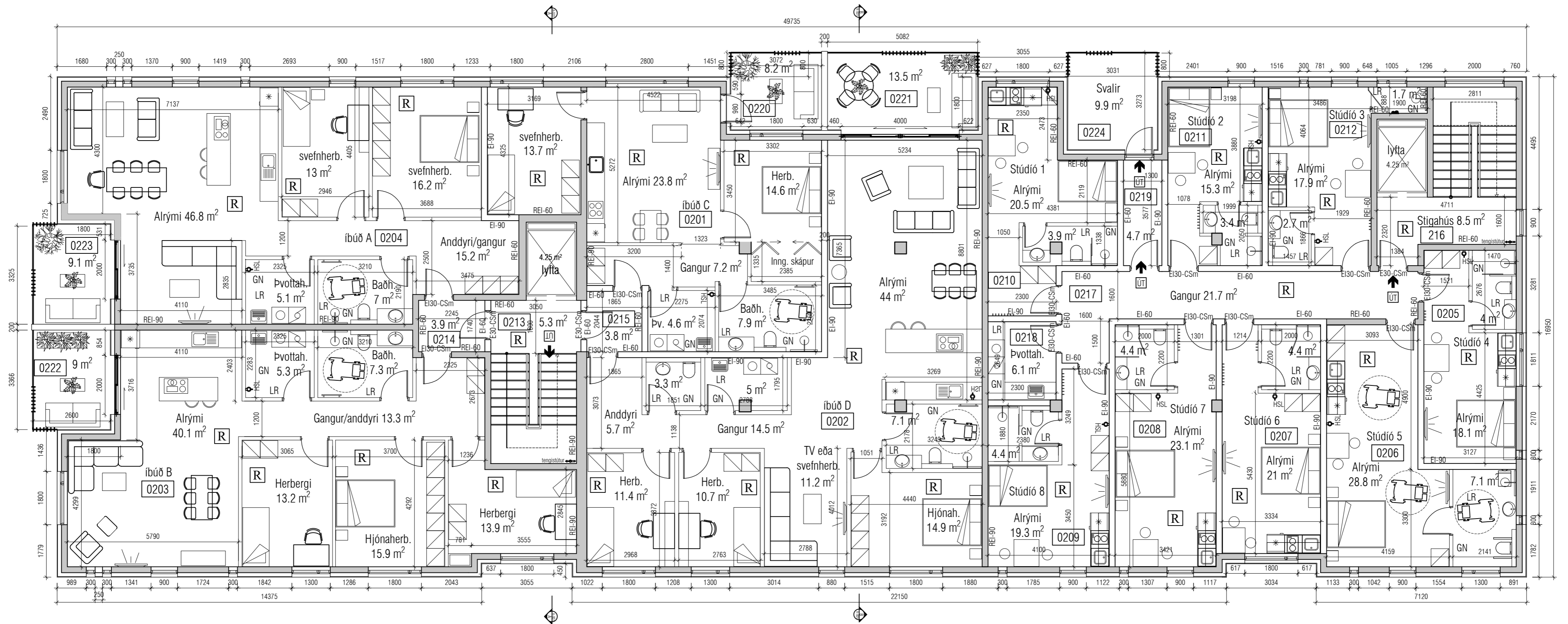
2. Hæð - 1:100
